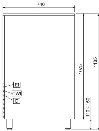
Zij aanzicht
